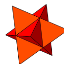
2 Tetraeder (Feuer)
